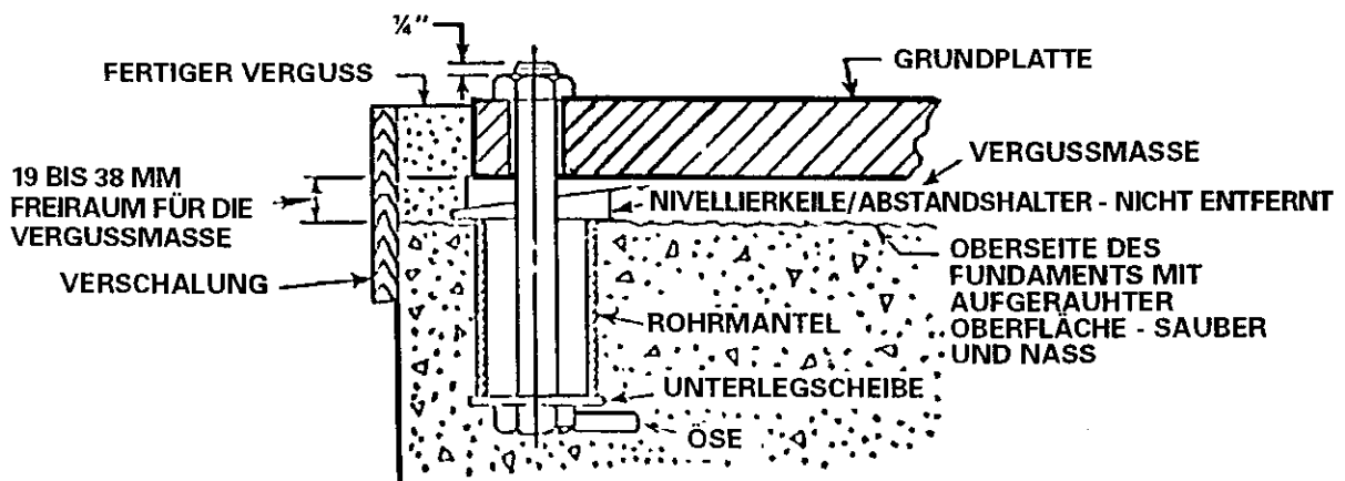
ABB. 3 TYPISCHES FUNDAMENTBOLZEN-DESIGN
